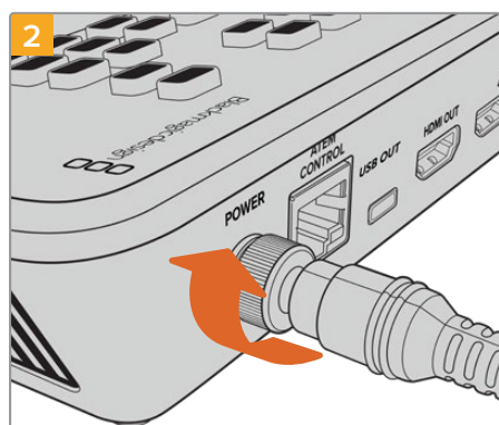
Sichern Sie die Kabelverbindung zum ATEM Mini, indem Sie den Verbinder am Gerät festziehen
