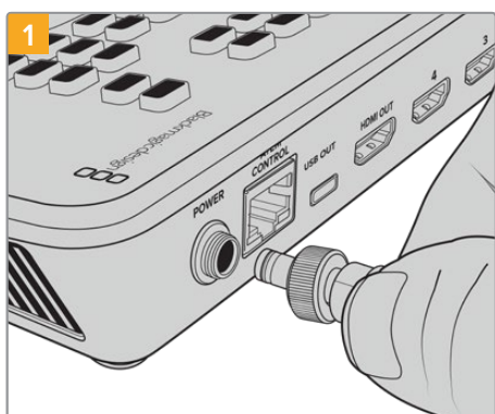
Stecken Sie das mitgelieferte Kabel in die Strombuchse am ATEM Mini
