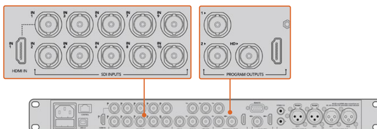
Anschluss einer Blackmagic Studio Camera an einen beliebigen SDI-Eingang Ihres ATEM Mixers
