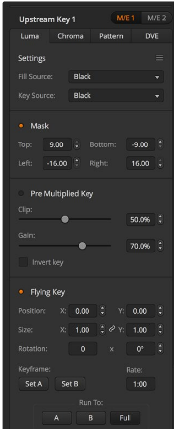
Luma Key Ayarları
