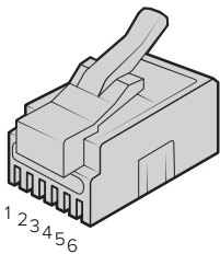
ATEM Constellation 8K의 PTZ 원격 연결을 위한 RJ12 핀 배치도
