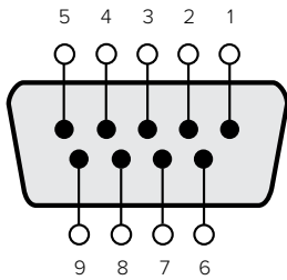
RS-422 PTZ 핀 배치도
